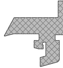
043198 Dichtungsprofil für Nullschwelle Joint pour seuil VE = 25 lfm
